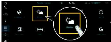
图 12：天气
