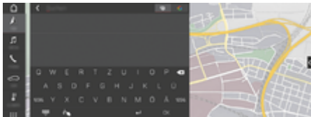
图 5: 查找工具
